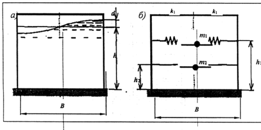
Рис.П.5.1. Моделирование резервуара с жидкостью:
